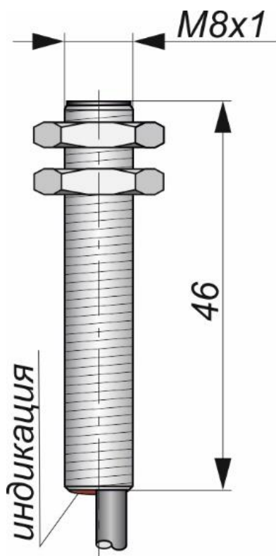
Габаритный чертеж
