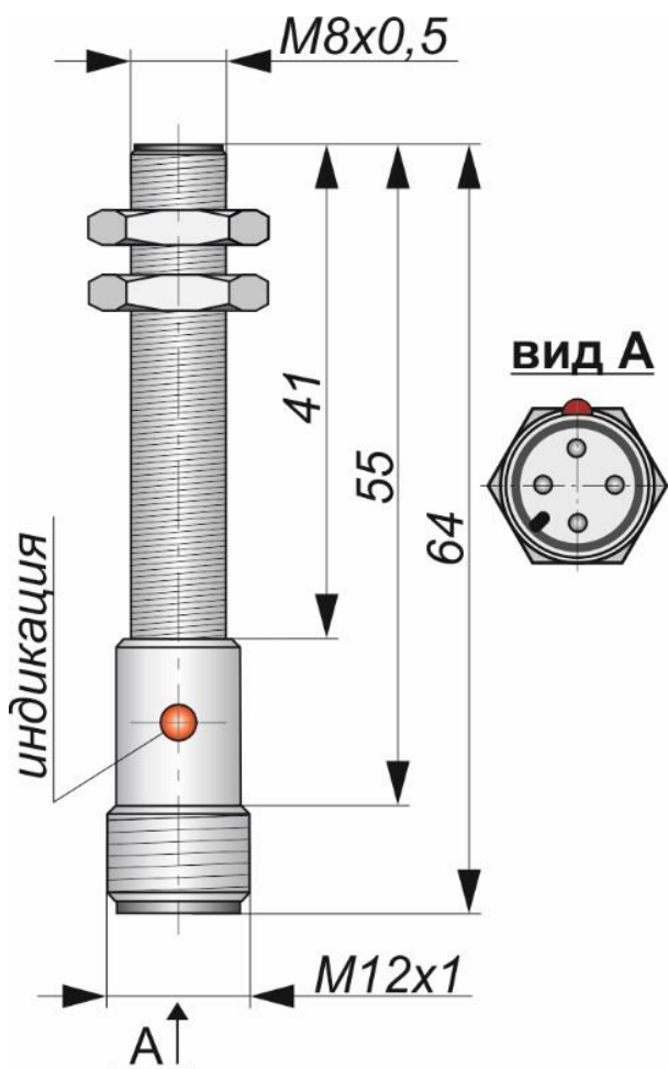
Габаритный чертеж
