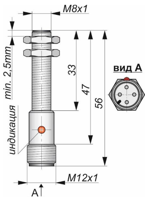
Габаритный чертеж
