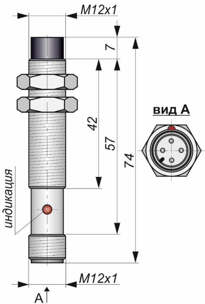
Габаритный чертеж
