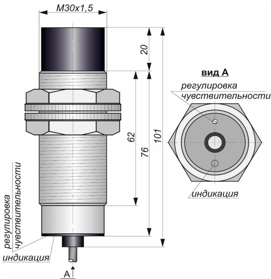
Габаритный чертеж
