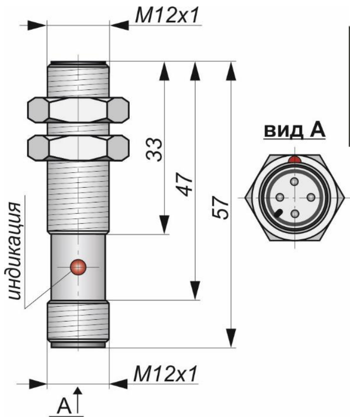
Габаритный чертеж
