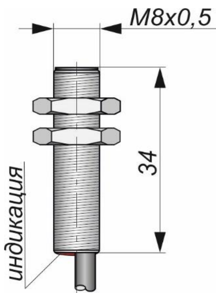
Габаритный чертеж
